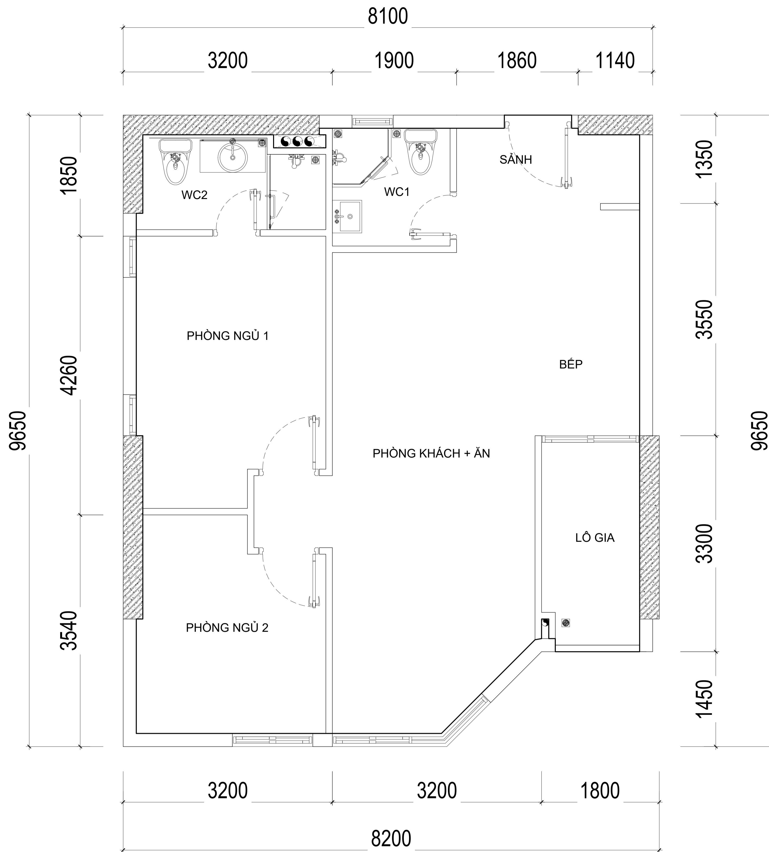
MẶT BẰNG CĂN HỘ SỐ 08
